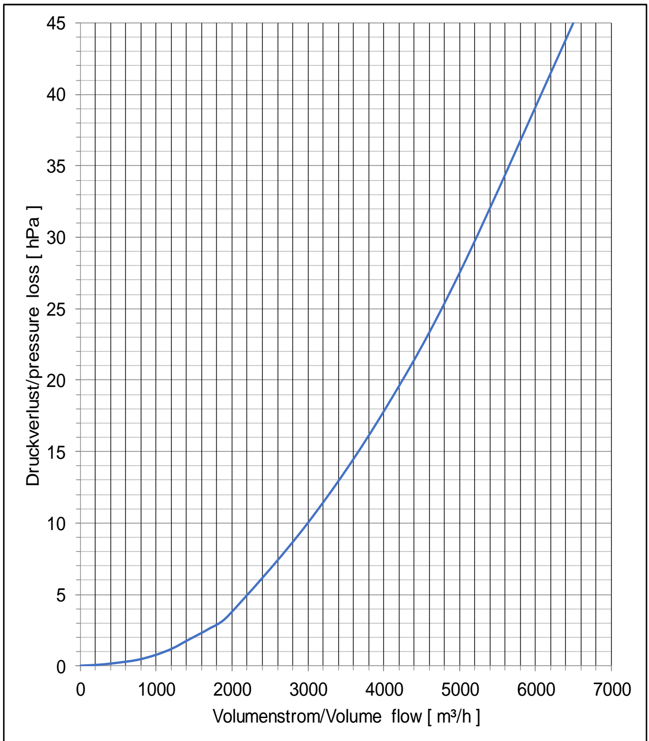
Bild 2: Druckverlust Medium Luft p_0 = 1005 \text{ mbar} , T_0 = 282\text{K} , Dichte = 1,241 \text{ kg/m}^3
