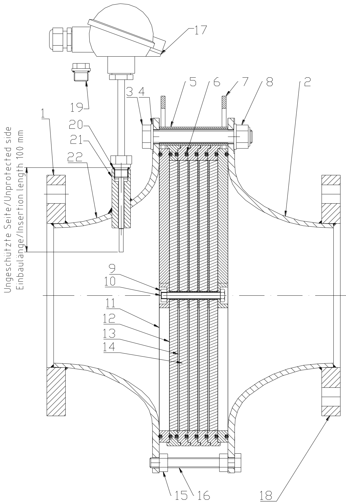
Bild 1 Konstruktion
